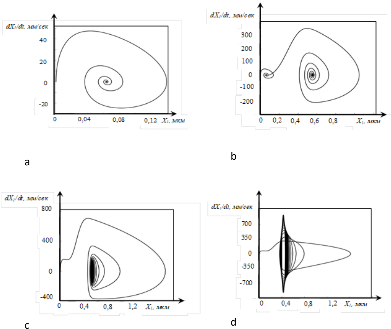
Рис. 3. Преобразование проекций фазовых траекторий на плоскость X_1 - dX_1/dt в зависимости от параметра T_w интегрального оператора и скорости относительного скольжения V_0 : а - T_w = 1 \text{ сек} , V_0 = 0,05 \text{ м/сек} ; б - T_w = 0,5 \text{ сек} , V_0 = 0,2 \text{ м/сек} ; в - T_w = 0,1 \text{ сек} , V_0 = 1 \text{ м/сек} ; д - T_w = 0,01 \text{ сек} , V_0 = 2 \text{ м/сек} .
