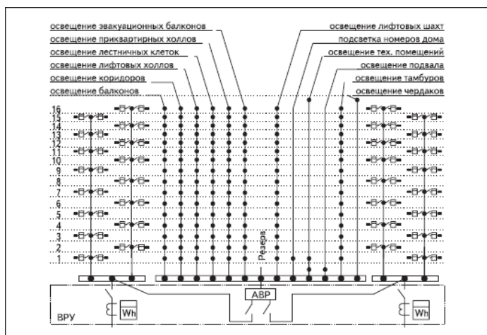
Рис. 3. Принципиальная однолинейная схема электроснабжения 2-подъездного 16-этажного жилого дома
