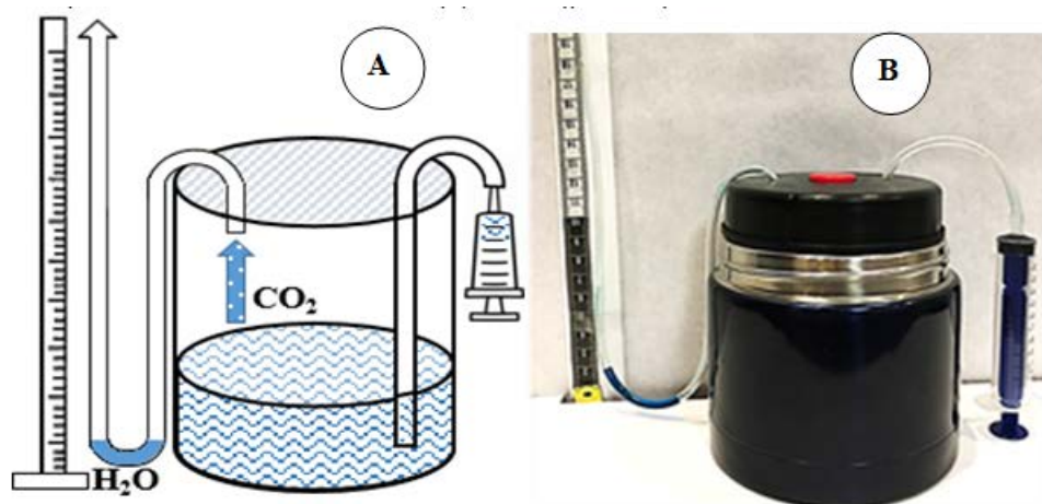
Рисунок 1. Схема (А) и фото (В) конструкции для проведения опыта
